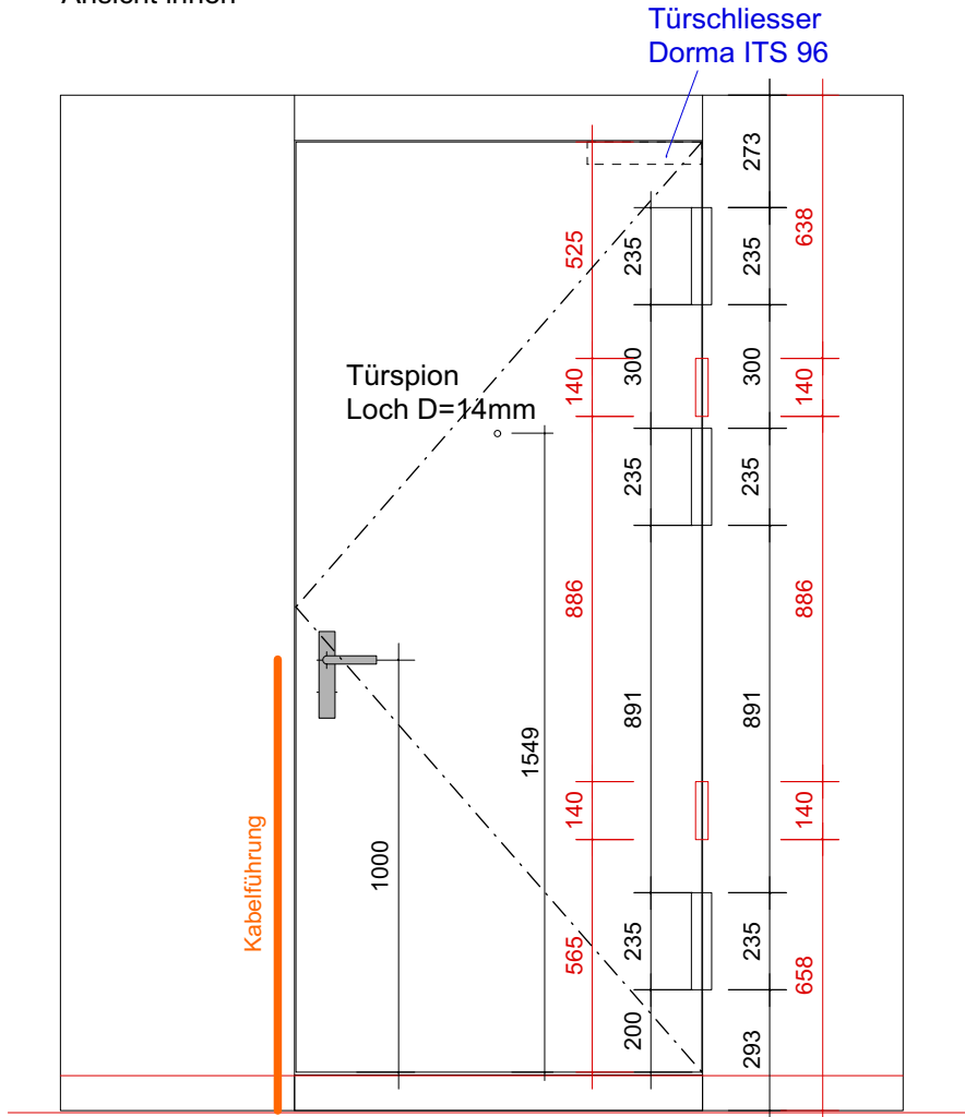
Ansicht innen
